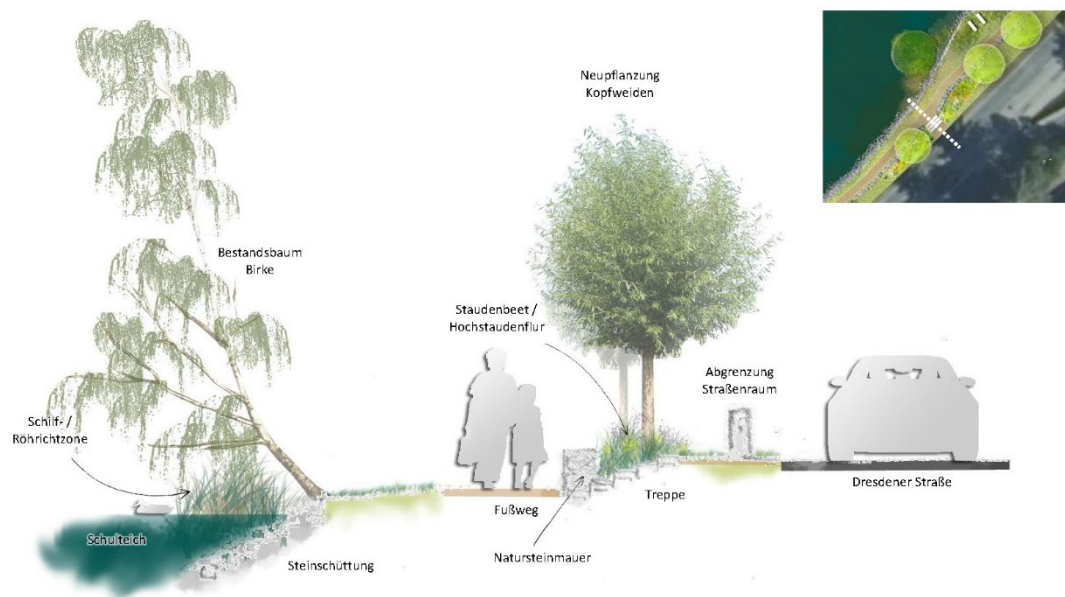
Abb. 15: Schnittansicht Nordufer Konzeption Vorentwurf, neuland
