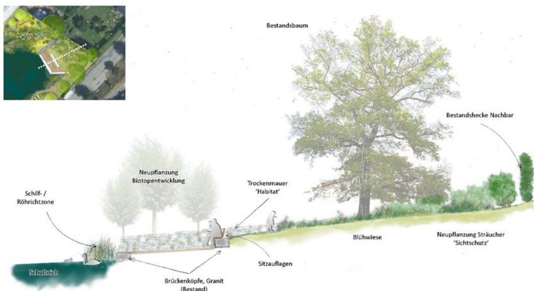
Abb. 14: Schnittansicht Nordufer Konzeption Vorentwurf, neuland
